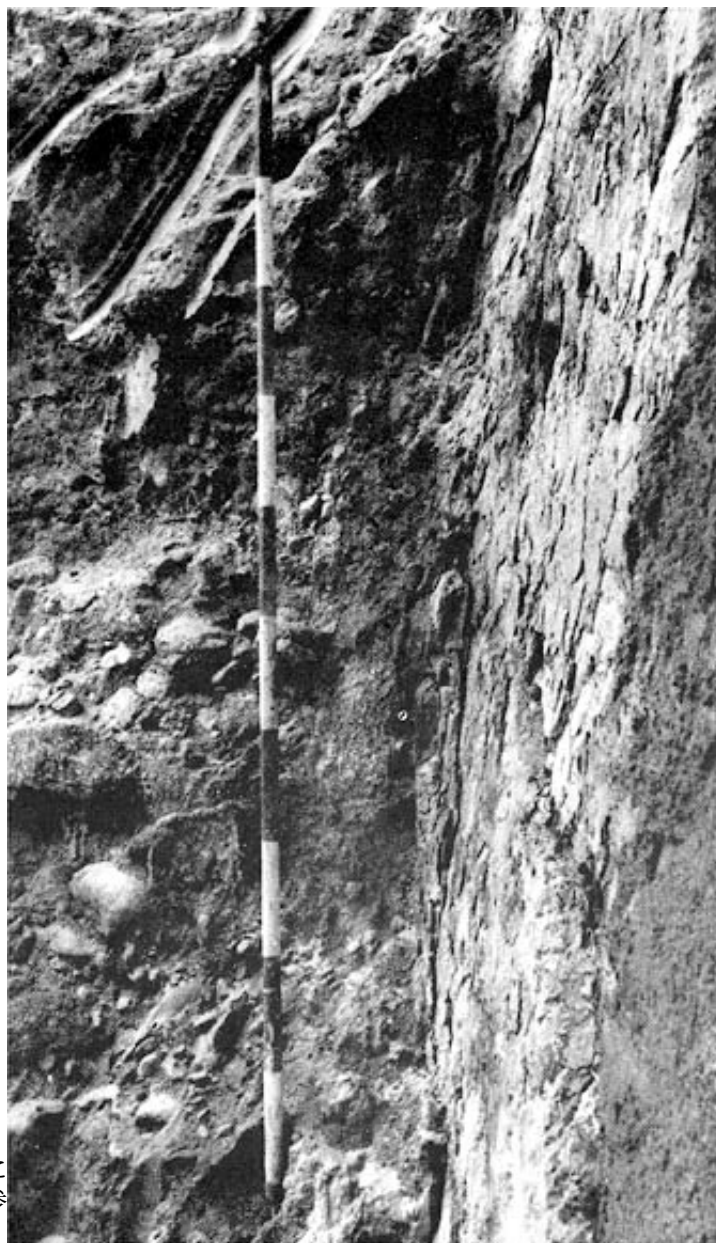
新神戸駅敷地にあらわれた諏訪山断層面、断層にひきづられて石が斜めに立っている。47ページ参照（昭45撮）
