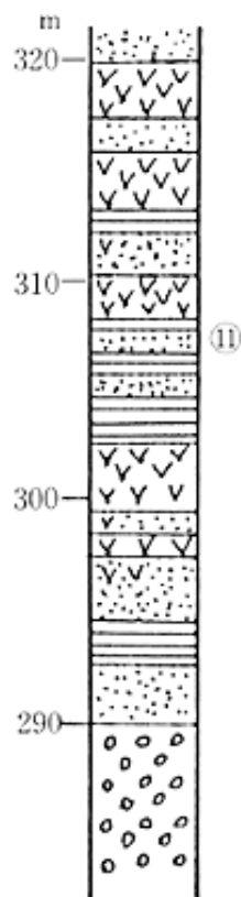
▲発見地点 北区山田町藍那 の柱状図
