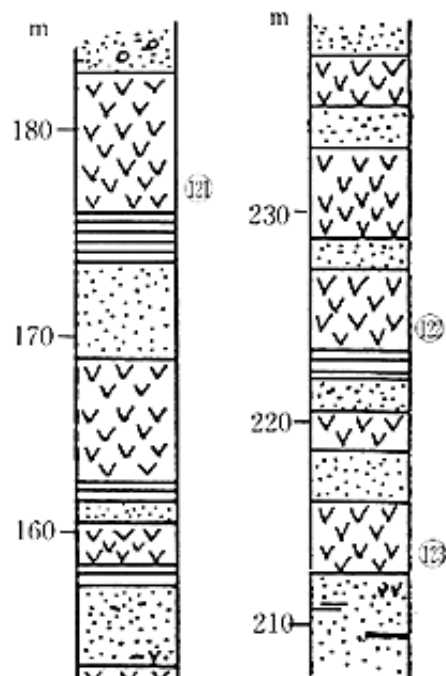
▲発見場所 兵庫区鶴台 の柱状図
