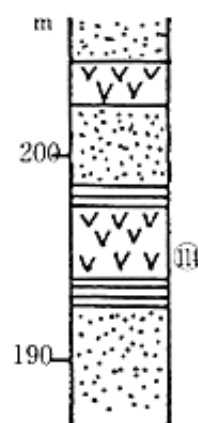
▲発見場所 北区山田町 の柱状図
