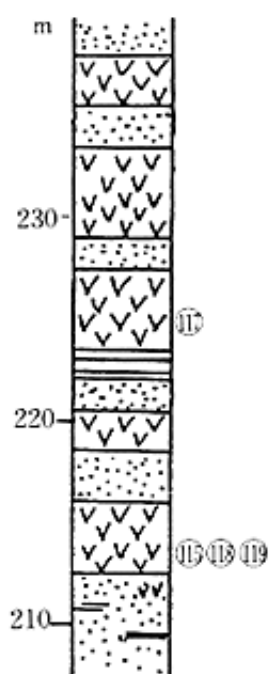
▲発見場所 兵庫区鶴台 の柱状図
