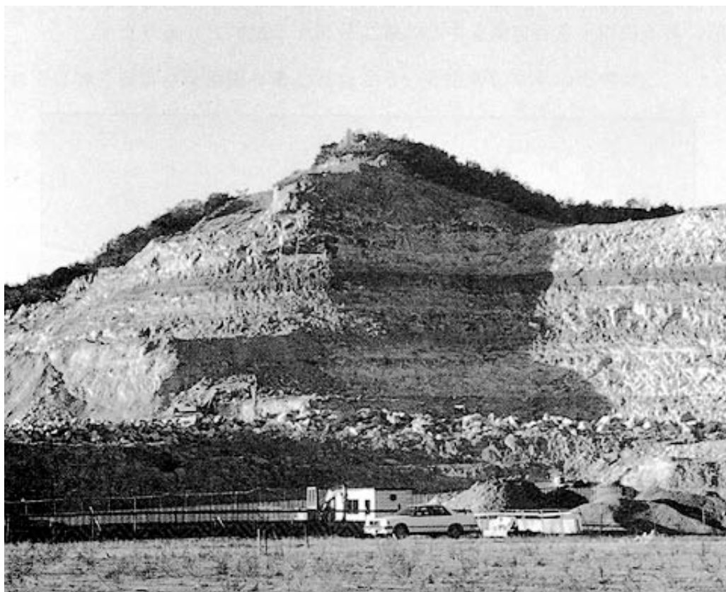
▲開発工事であらわれた神戸層群の水平な地層 (須磨区総合運動公園北、昭和62年撮影)
