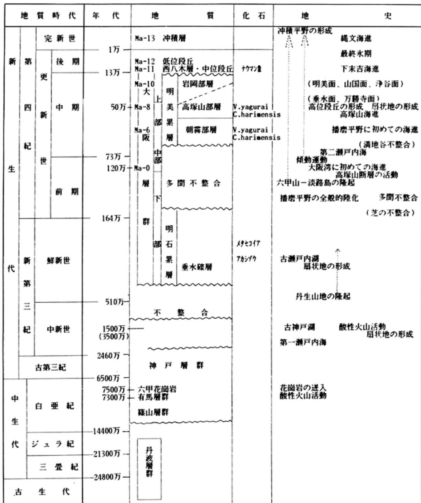
図56 播磨平野の地層と歴史
